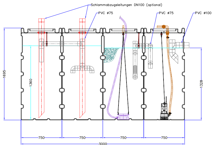
KELLERCHEN® 6 EW - Schnitt BB
