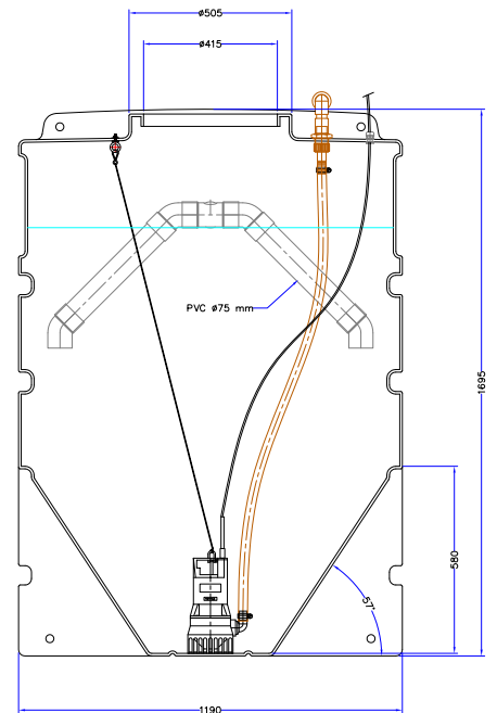
KELLERCHEN® 6 EW - Schnitt CC
