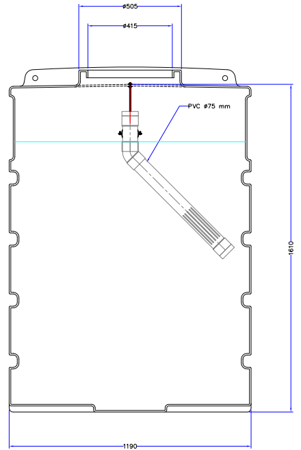
KELLERCHEN® 6 EW - Schnitt DD
