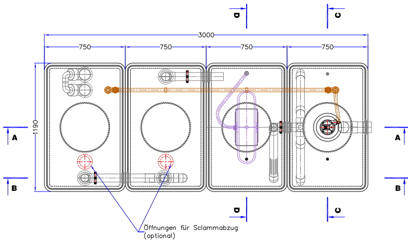
KELLERCHEN® 6 EW - Draufsicht
