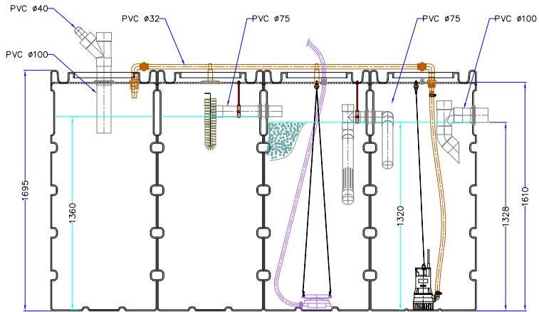
KELLERCHEN® 6 EW - Schnitt AA
